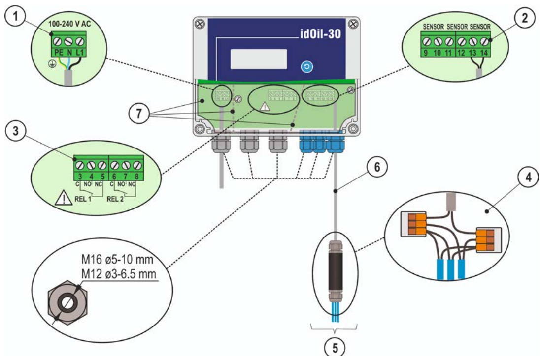
Rysunek 15. Podłączenie za pomocą trójczynnikowego złącza kablowego
