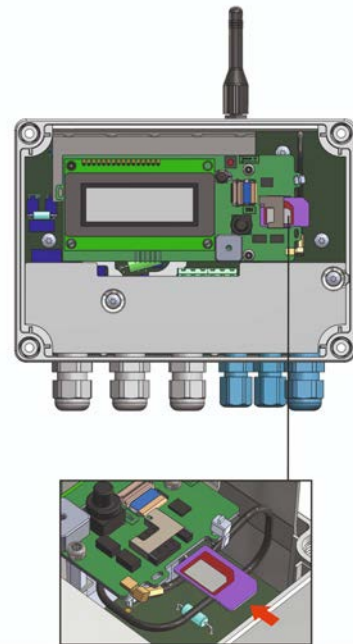
Rysunek 22. Instalowanie karty SIM
