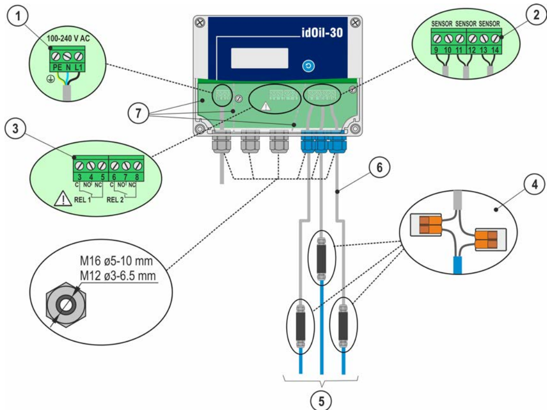
Rysunek 13. Podłączenie za pomocą jednoczujnikowego złącza kablowego
