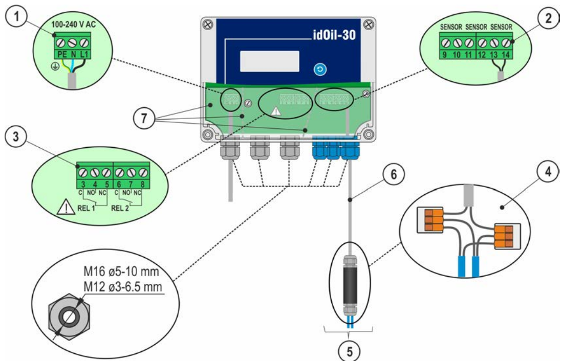
Rysunek 14. Podłączenie za pomocą dwuczynnikowego złącza kablowego
