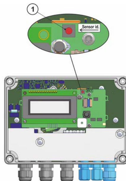
Rysunek 18. Przycisk identyfikacji czujników.
