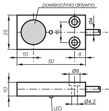
Rys. 22 - obudowa plastikowa P4
