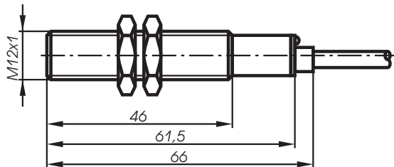
Rys. 7 - obudowa typu M12 A0
