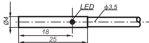
Rys. 2 - obudowa typu H4 A0
