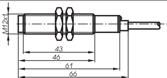
Rys. 9 - obudowa typu M12 A1
