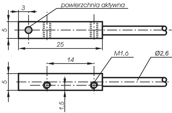
Rys. 21 - obudowa metalowa Q5
