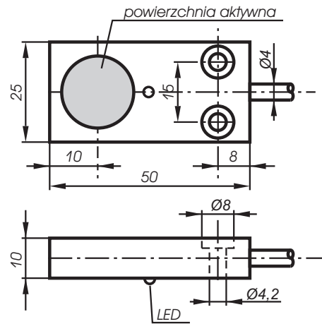
Rys. 22 - obudowa plastikowa P4
