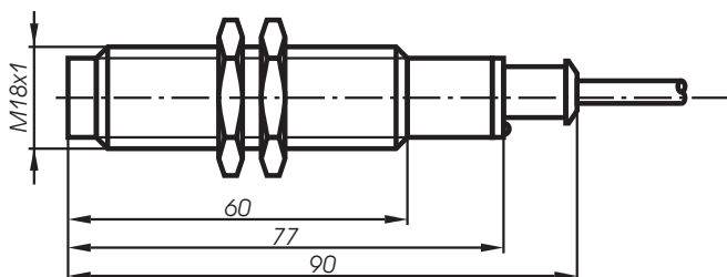
Rys. 13 - obudowa typu M18 A1
