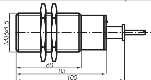
Rys. 19 - obudowa typu M36 A0
