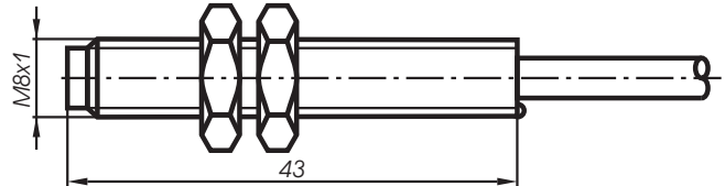
Rys. 6 - obudowa typu M8 A1
