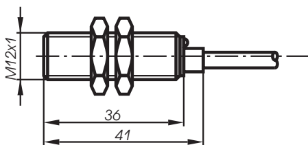
Rys. 8 - obudowa typu M12 A0 K
