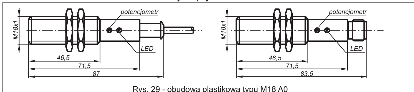
Rys. 29 - obudowa plastikowa typu M18 A0
