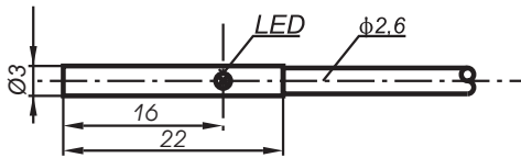
Rys. 1 - obudowa typu H3 A0
