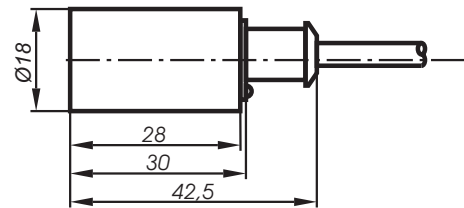
Rys. 25 - obudowa plastikowa P7
