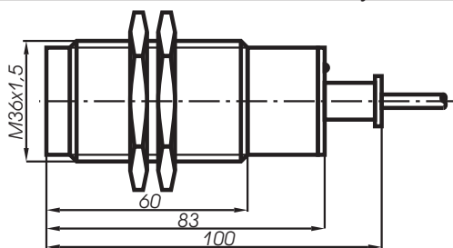
Rys. 20 - obudowa typu M36 A1
