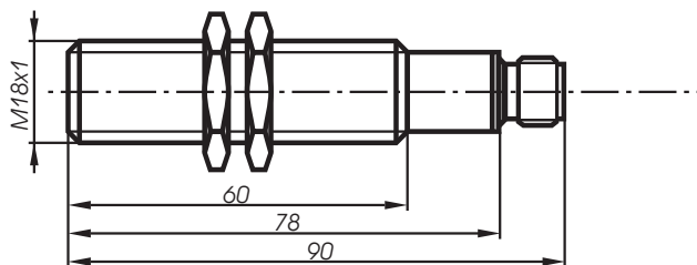
Rys. 11 - obudowa typu M18 A0
