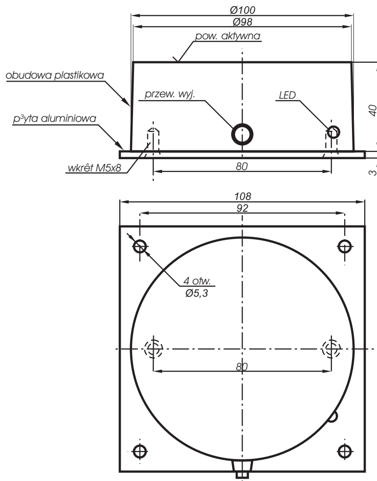
Rys. 27 obudowa typu P2
