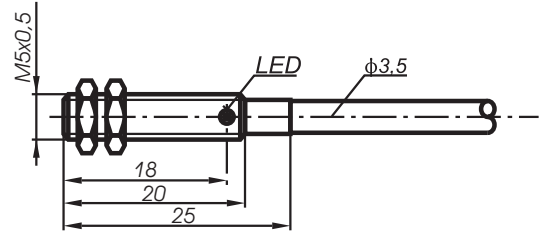
Rys. 4 - obudowa typu M5 A0
