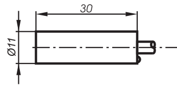
Rys. 24 - obudowa plastikowa P6
