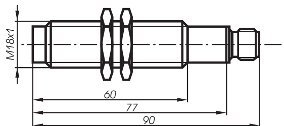
Rys. 13 - obudowa typu M18 A1
