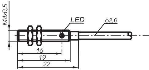
Rys. 3 - obudowa typu M4 A0
