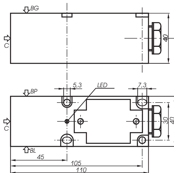
Rys. 28 obudowa plastikowa typu X
